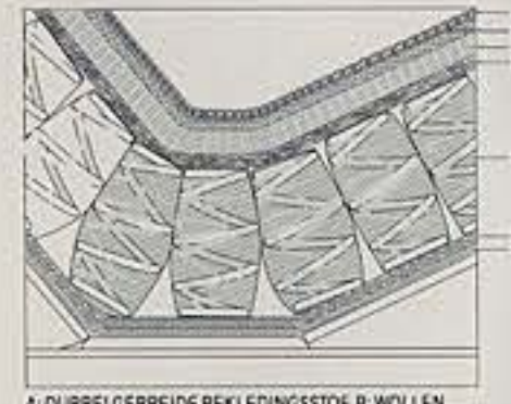
A: DUBBELGEBREIDE BEKLEDINGSSTOF, B: WOLLEN AFDEKLAAG, C: VERWARMINGSSET, D: COMFORT LAAG, E: ECOCEL, F: AFDEKLAAG PAARDEHAAR, G: TONVORMIGE POCKETVEREN, H: SUPPORTLAAG, I: VENTILATIEBODEM.
