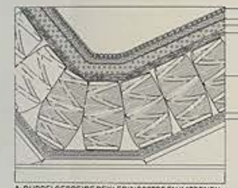
A: DUBBELGEBREIDE BEKLEDINGSSTOF EN KATOENEN AFDEKLAAG, B: VERWARMINGSSET, C: COMFORT LAAG, E: ECOCEL, D: AFDEKLAAG PAARDEHAAR, E: TONVORMIGE POCKETVEREN, F: SUPPORTLAAG, G: VENTILATIEBODEM.
